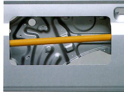
サイドアビーム(全車に標準) 写真は機能説明のために着色したものです。
