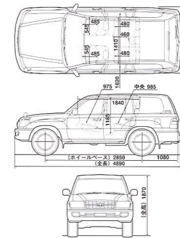
WAGON VX
